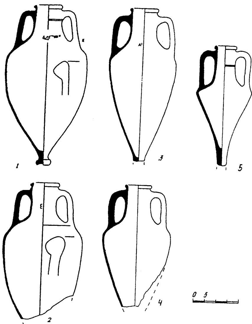
Рис.2 Клеймённые амфоры Батилла из раскопок поселения Панское I. (Чертежи по С. Монахову и А. Щеглову)
